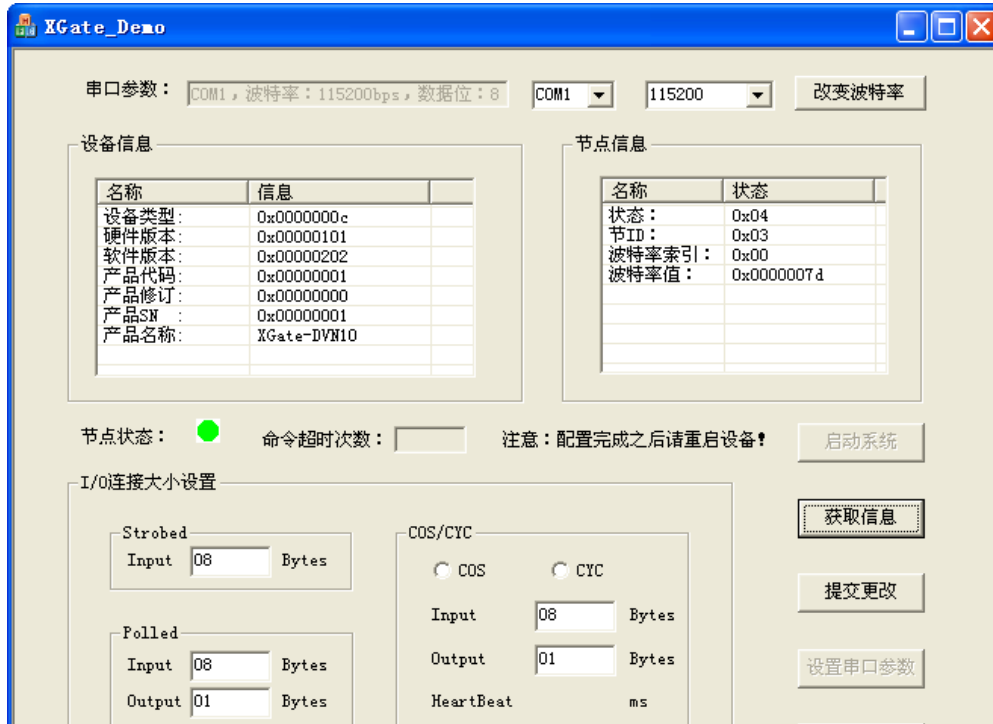
图 2.8 XGate 配置 Demo 软件
