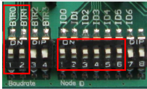
图 2.6 拨码开关设置
