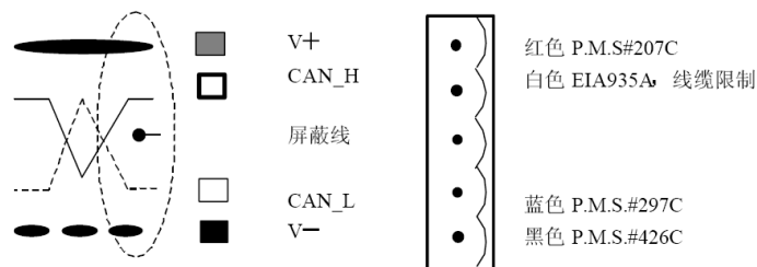
图 2.5 开放式连接器连接示意图
