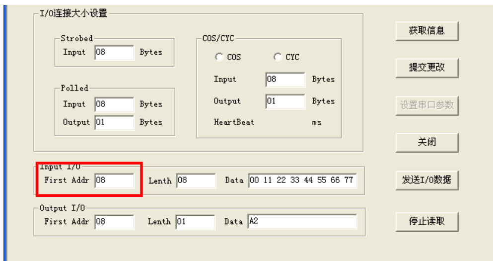
图 2.9 XGate 配置 Demo 软件
