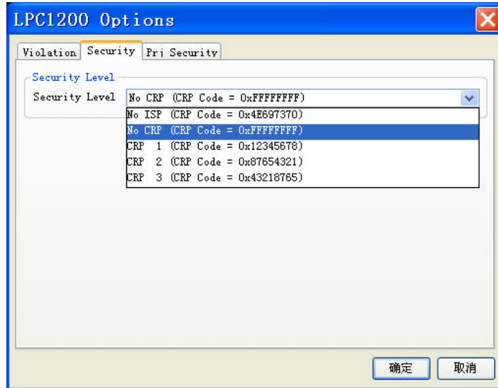
图 3.6 配置 LPC1227 的加密级别
