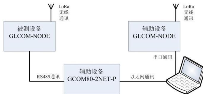
图 1 试验配置示意图
