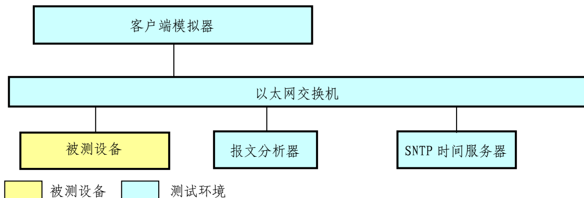
图 3.1 测试系统组成
