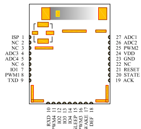
引脚分布图
