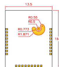
BOTTOM视图
