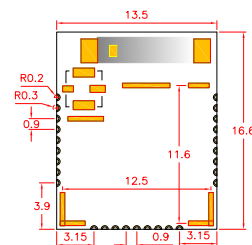
TOP视图
